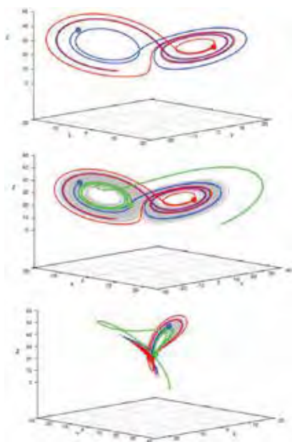
De vlinder van Lorenz
