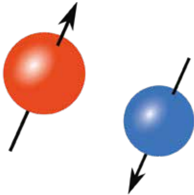
Twee elektronen spin's
